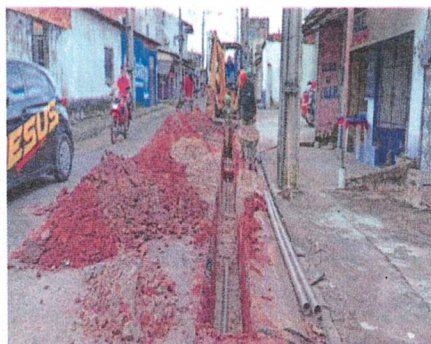
Assentamento de Redes de Água no Bairro do Bengui – Município de Belém
