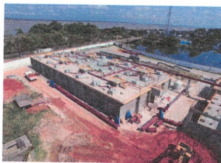
Estação de Tratamento de Esgotamento Sanitário ETE-UNA
