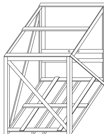
Engradado para transformadores de distribuição trifásicos.
