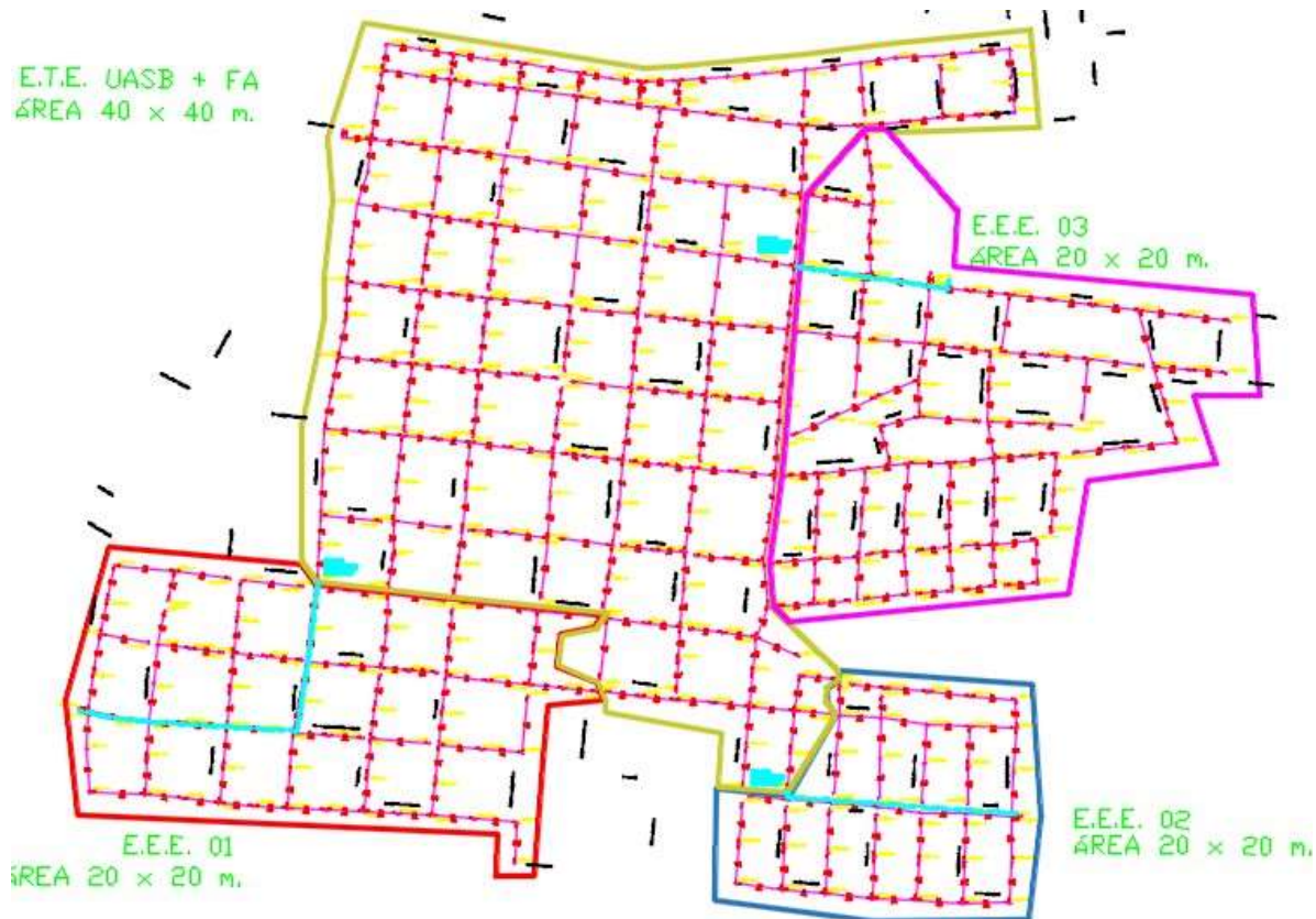
Figura 02 – Rede coletora proposta para o distrito de Alter do Chão.
