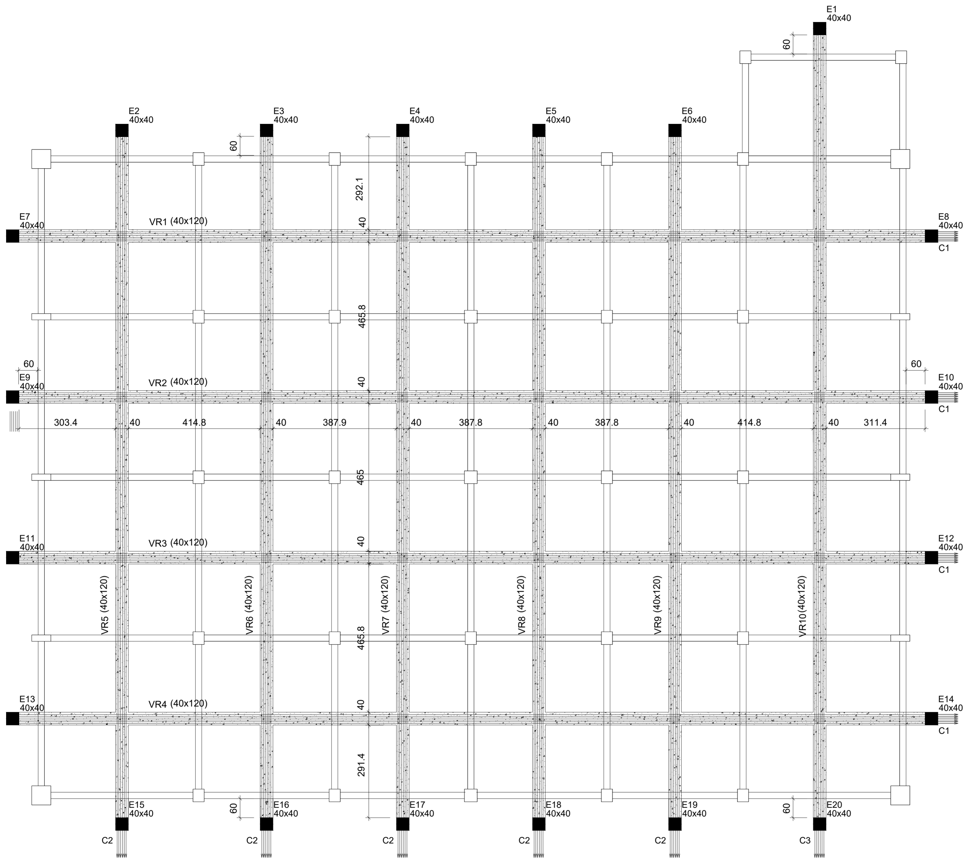
FORMA DAS VIGAS DE REFORÇO PROTENDIDAS ESCALA 1:50
