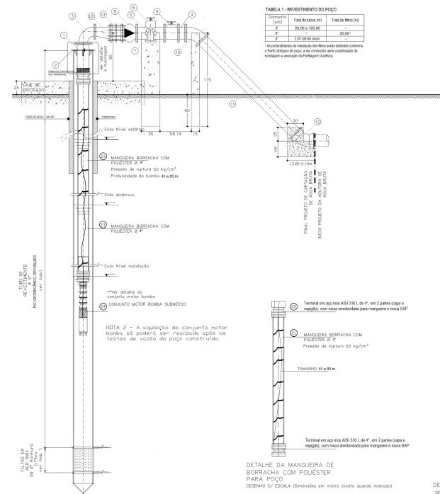
POÇO PROFUNDO - DETALHE DO BARRILETE VISTA EM ELEVAÇÃO DESENHO 5/ ESCALA (DIMENSÕES EM CENTÍMETRO EXCETO QUANDO INDICADO) ESCALA DE REFERÊNCIA 1:25
