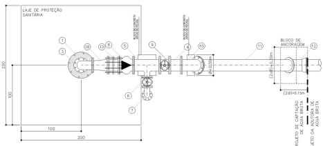
POÇO PROFUNDO - DETALHE DO BARRILETE PLANTA BAIXA DESENHO 5/ ESCALA (DIMENSÕES EM CENTÍMETRO EXCETO QUANDO INDICADO) ESCALA DE REFERÊNCIA 1:25
