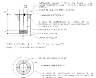
PEÇA ESPECIAL # 1 - VISTA EM ELEVAÇÃO ESCALA 1/125 (DIMENSÕES EM CENTÍMETRO)
