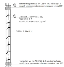
DETALHE DA MANGUEIRA DE BORRACHA COM FOLESTER PARA POÇO DESENHO 5/ ESCALA (DIMENSÕES EM METRO EXCETO QUANDO INDICADO)
