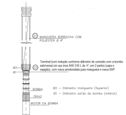
DETALHE - CONJUNTO MOTOR BOMBA DESENHO 5/ ESCALA (DIMENSÕES EM METRO EXCETO QUANDO INDICADO)
