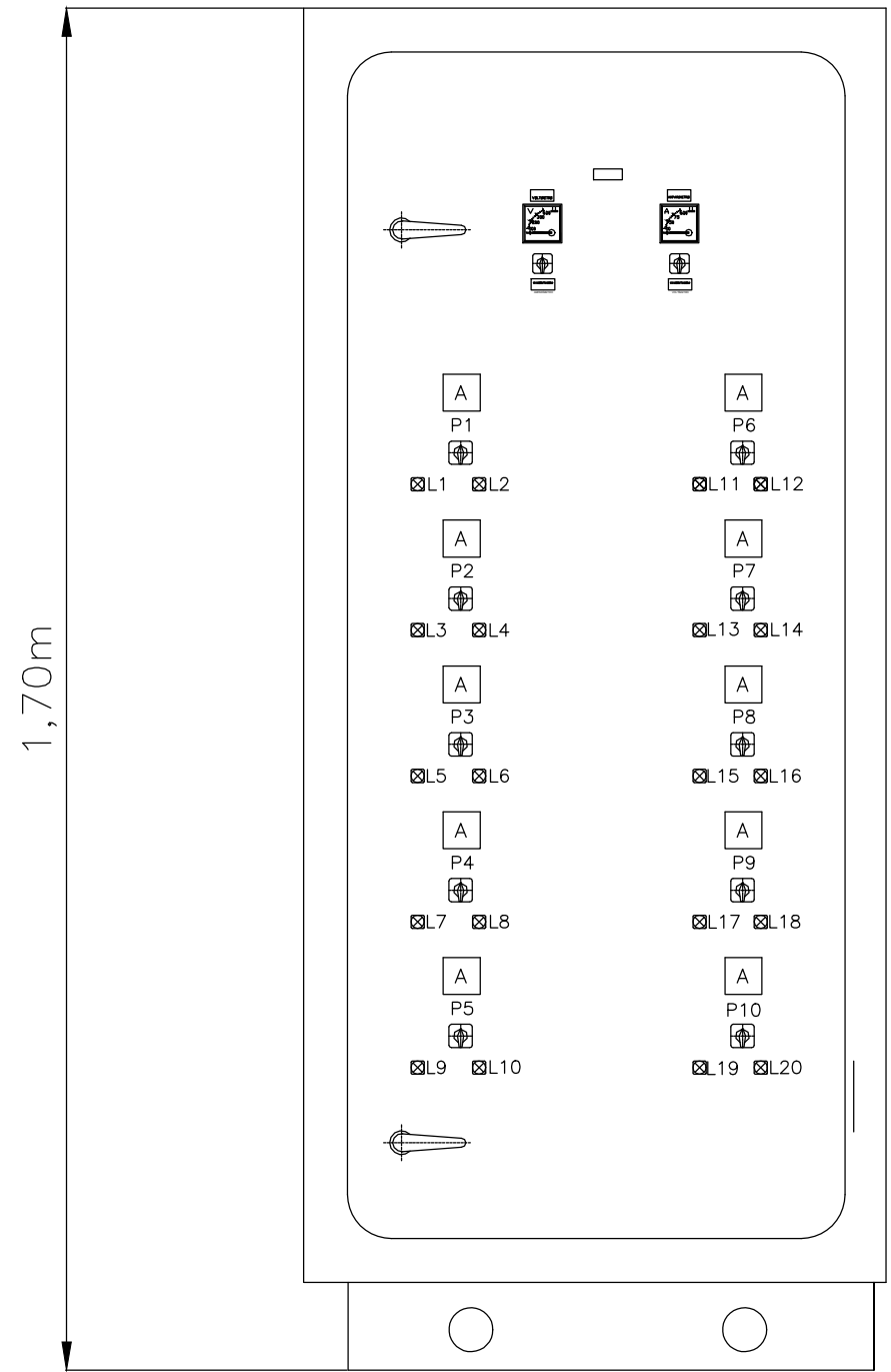
VISTA FRONTAL COM PORTA FECHADA DO CCM
