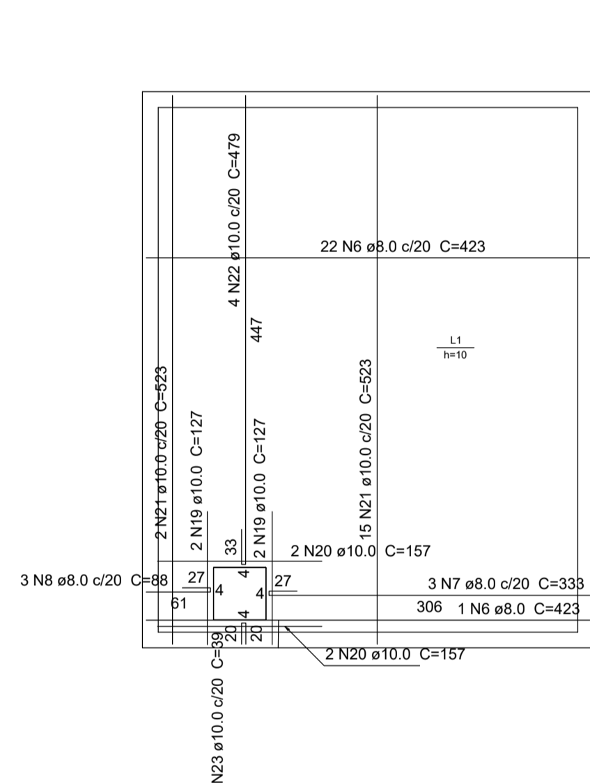
ARMAÇÃO POSITIVA DAS LAJES DE TAMPA ESC. 1:50
