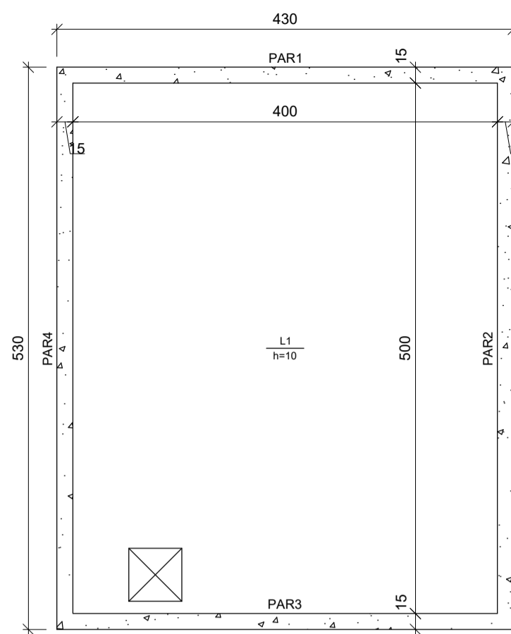
FORMA DA CISTERNA - TAMPA ESC. 1:50
