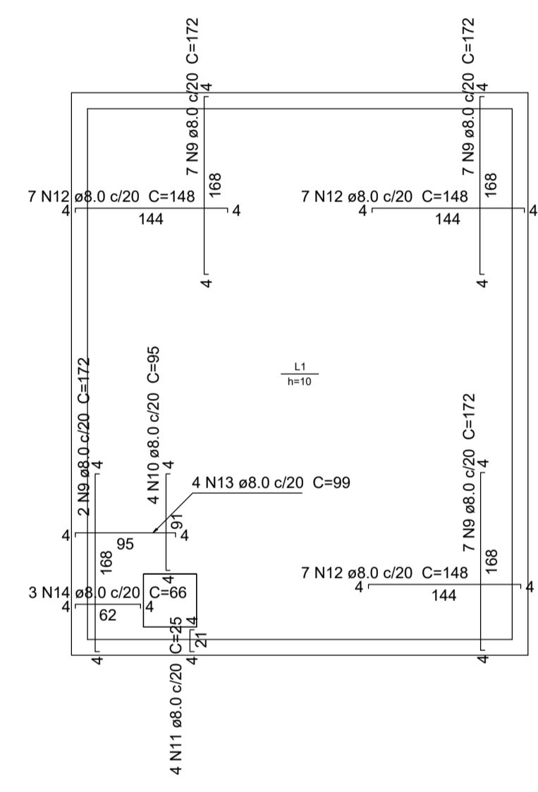
ARMAÇÃO NEGATIVA DAS LAJES DE TAMPA ESC. 1:50
