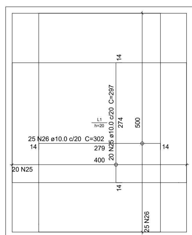
ARMAÇÃO NEGATIVA DAS LAJES DE FUNDO ESC. 1:50
