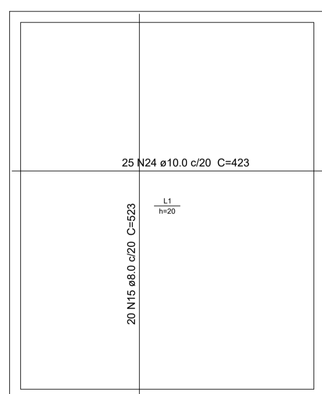
ARMAÇÃO POSITIVA DAS LAJES DE FUNDO ESC. 1:50
