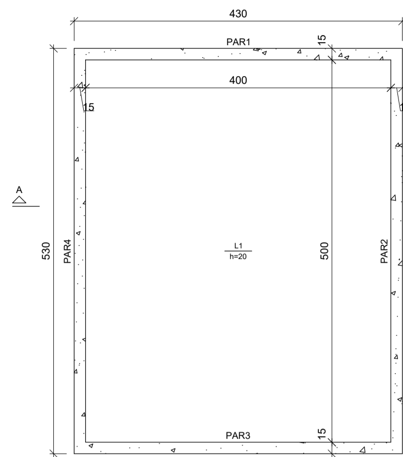
FORMA DA CISTERNA - FUNDO ESC. 1:50
