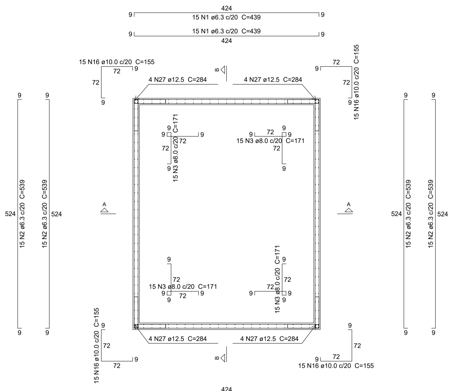
ARMAÇÃO EM PLANTA ESC. 1:50
