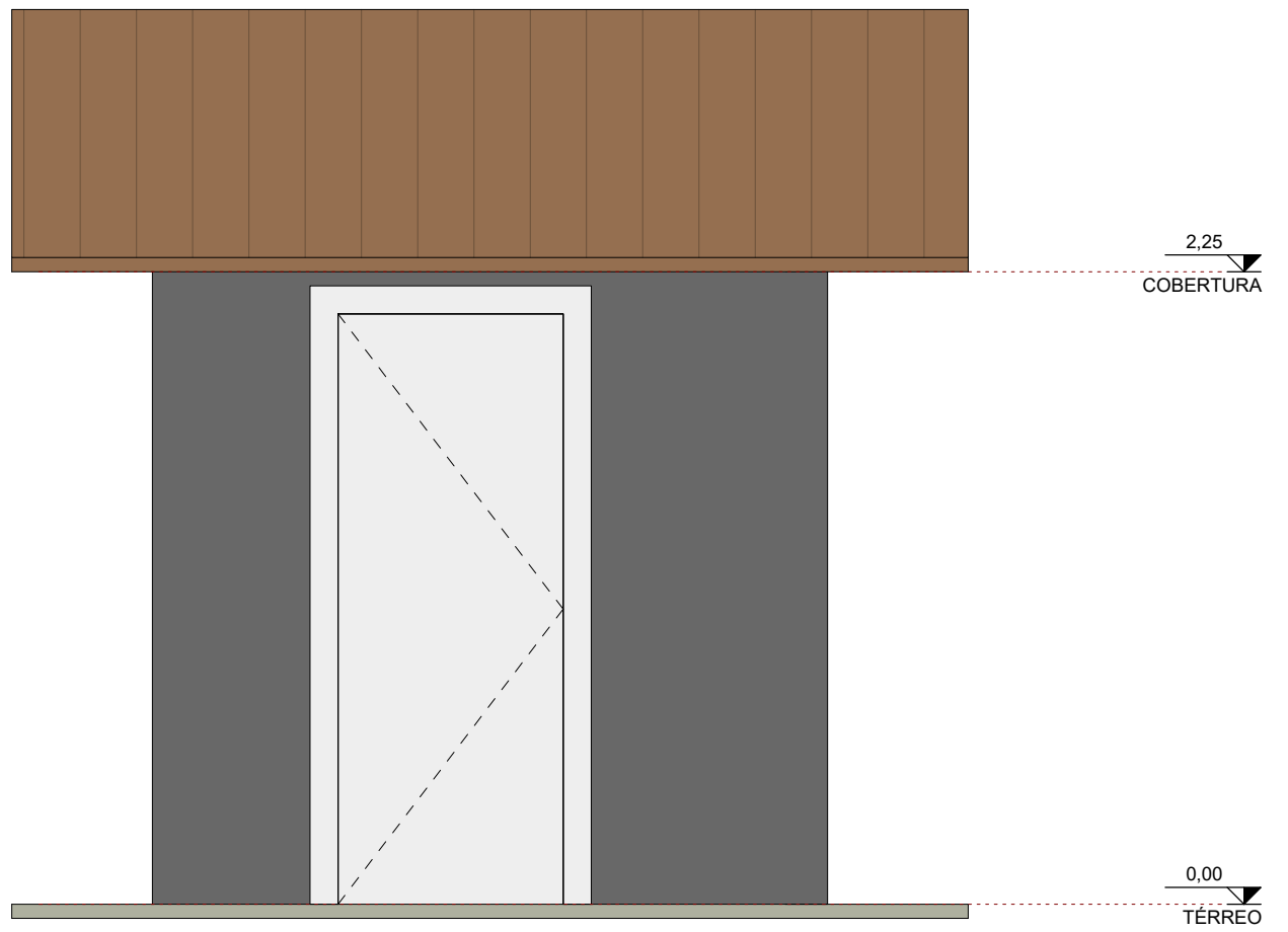
2 ELEVAÇÃO 01 ESCALA - 1 : 20
