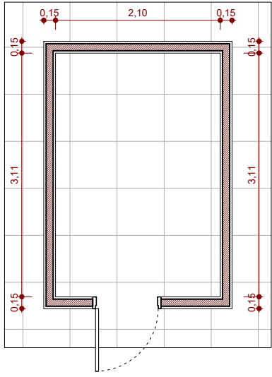
1 TÉRREO ESCALA - 1 : 50
