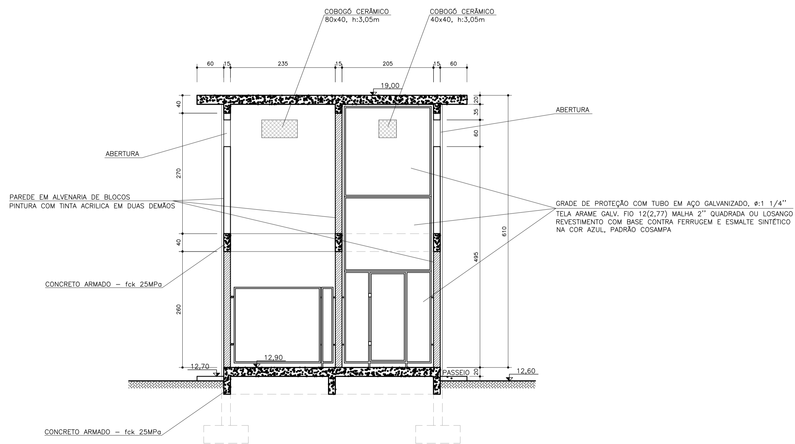
CORTE-A-A ESCALA 1/50
