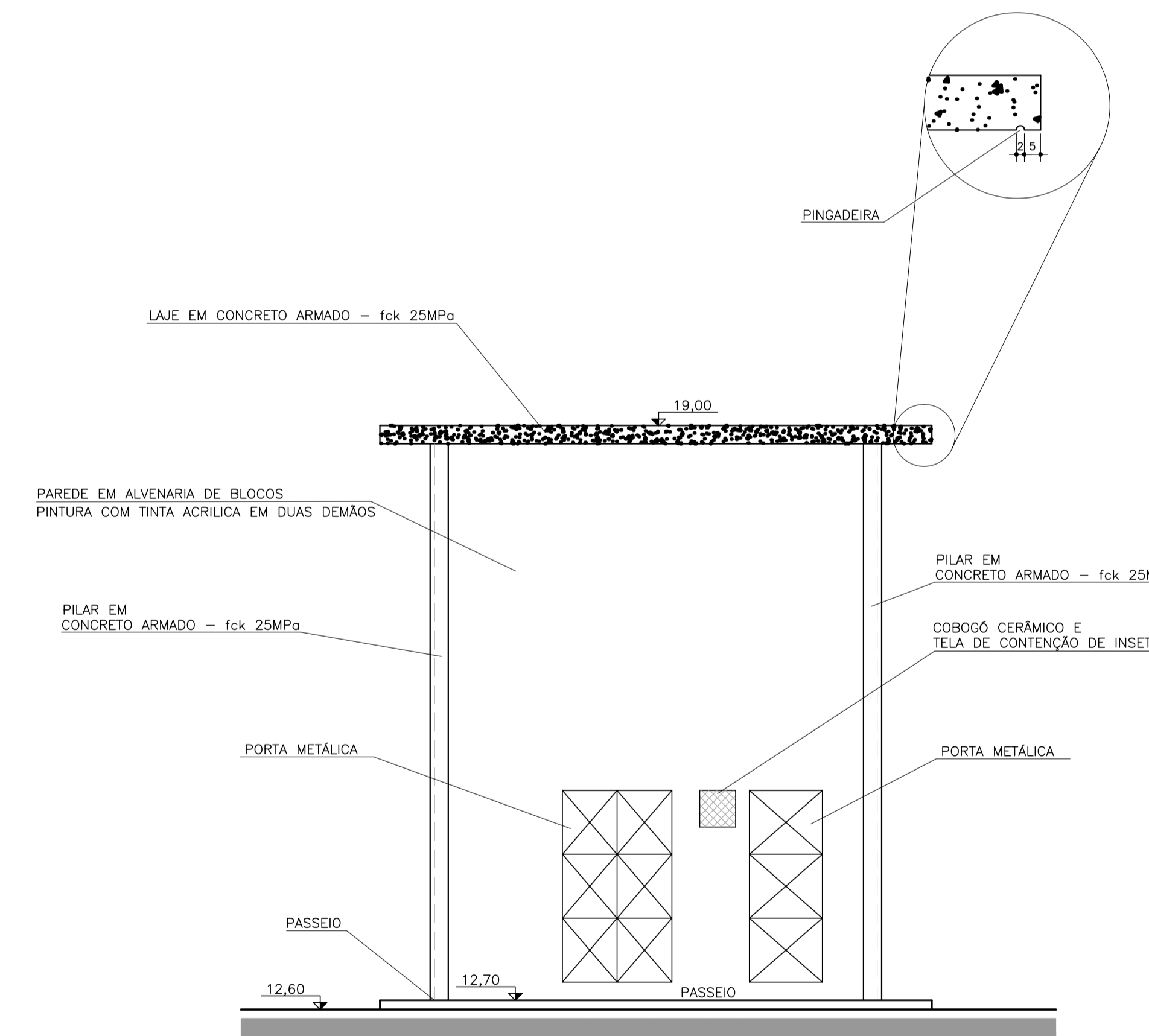
FACHADA ESCALA 1/50
