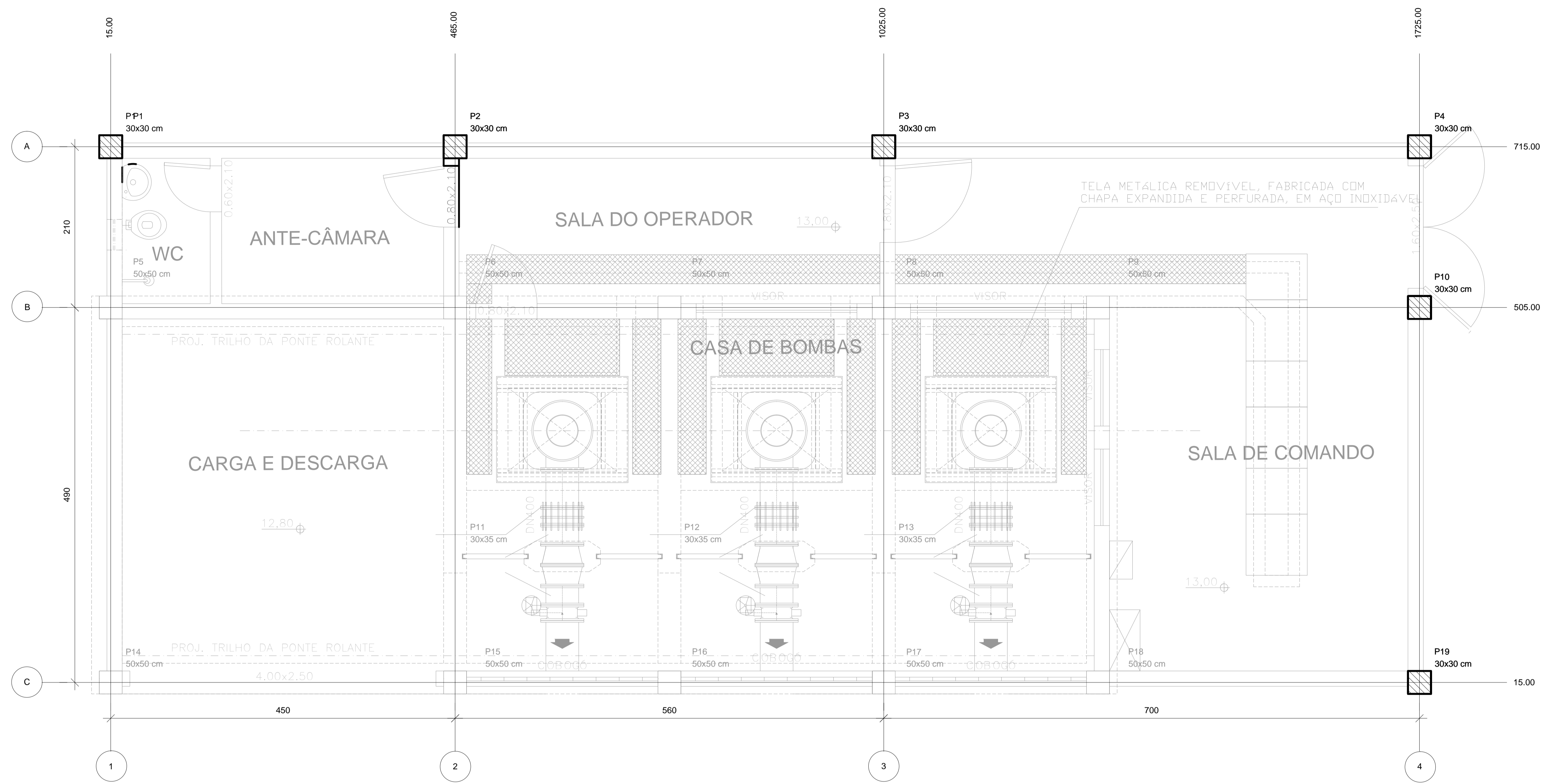
PLANTA DE LOCAÇÃO E CARGA DOS PILARES ESCALA 1:30
