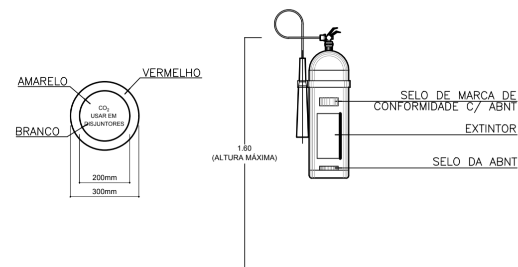
DETALHE DOS EXTINTORES S/ESCALA
