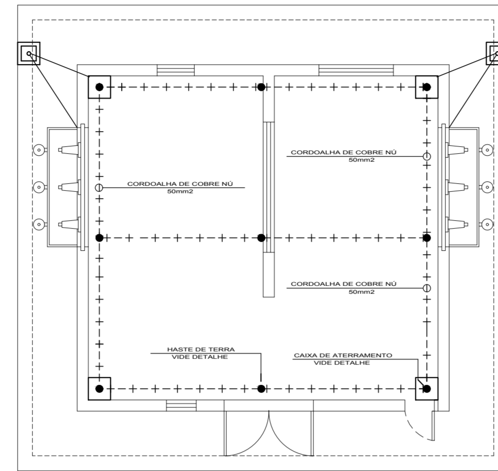
MALHA DE ATERRAMENTO
