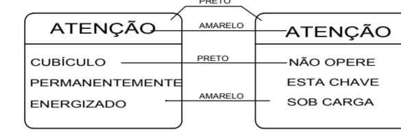
DETALHE DAS PLACAS DE ADVERTÊNCIAS S/ESCALA
