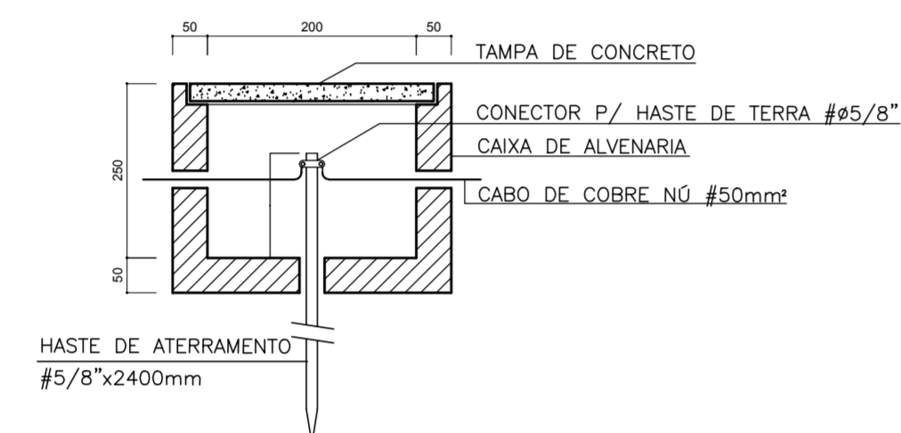
DET. CX DE ATERRAMENTO S/ESCALA
