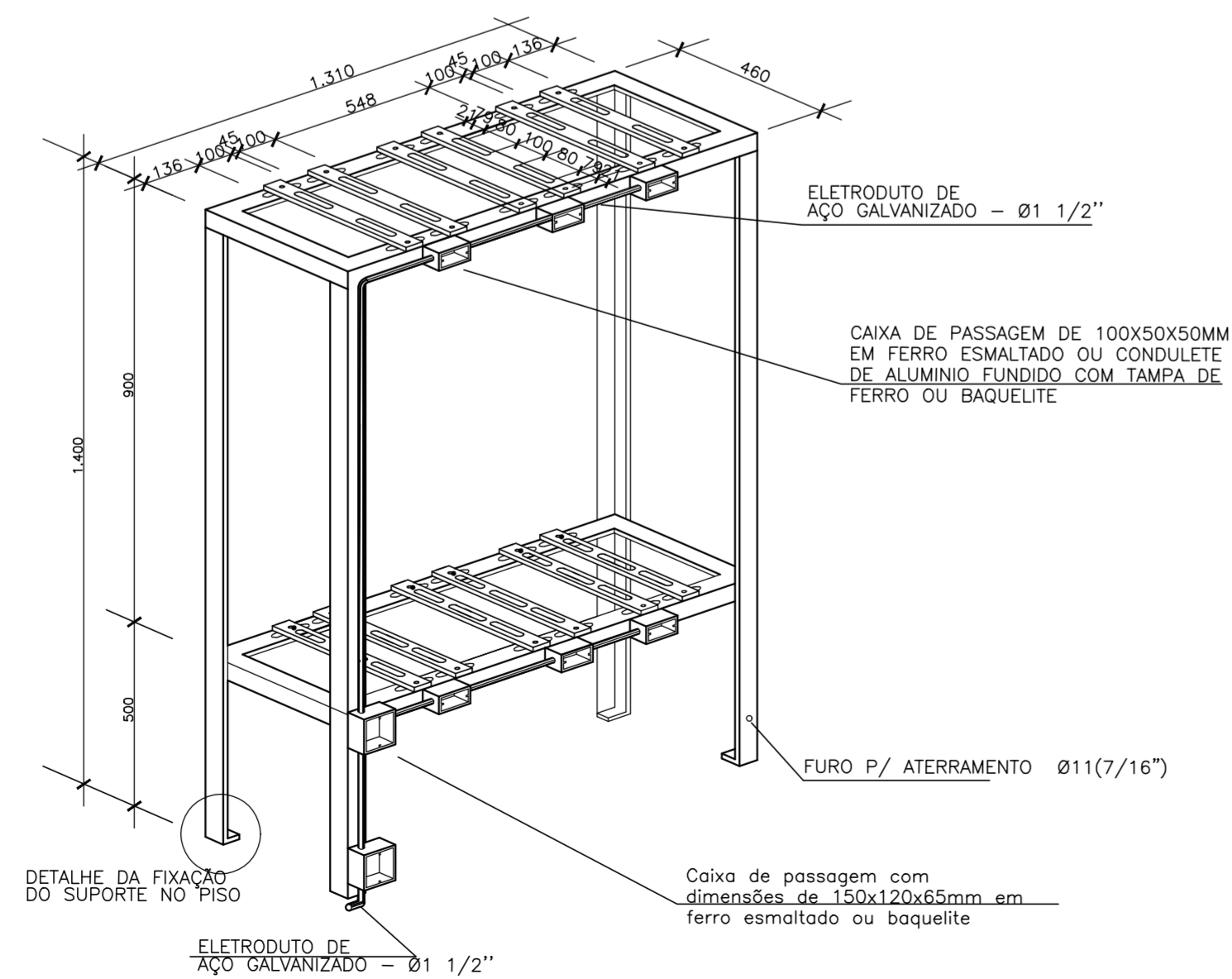
SUPORTE PARA T.P. E T.C. S/ESCALA
