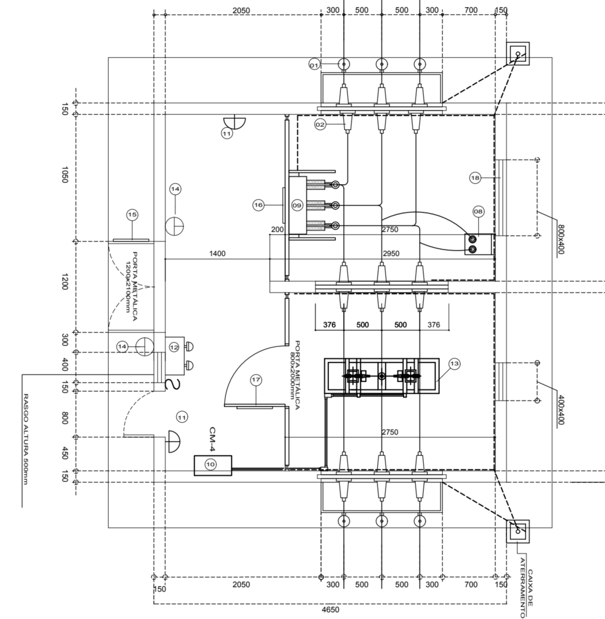
PLANTA BAIXA
