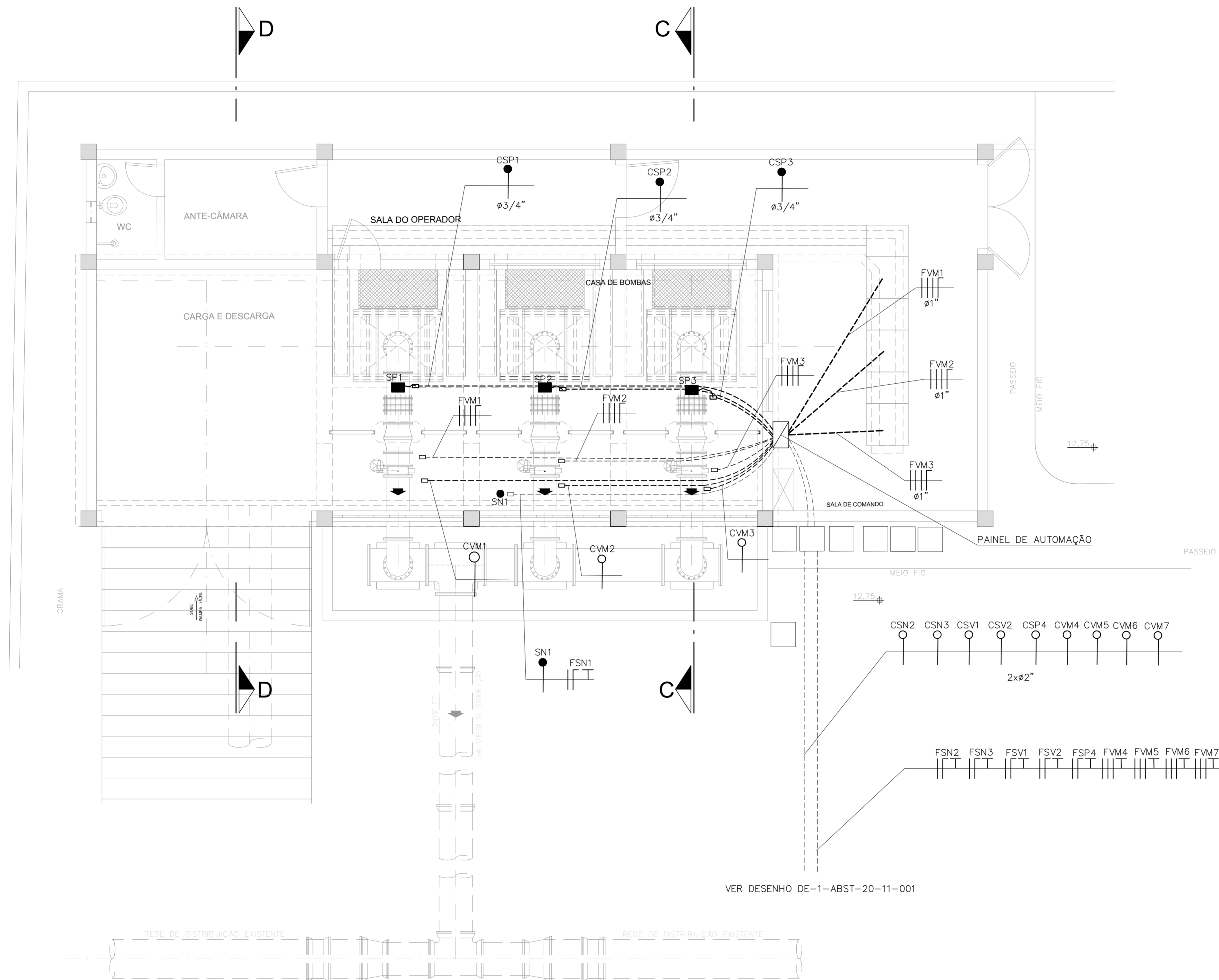
PLANTA BAIXA NO NÍVEL 13,00 ESCALA: 1/50
