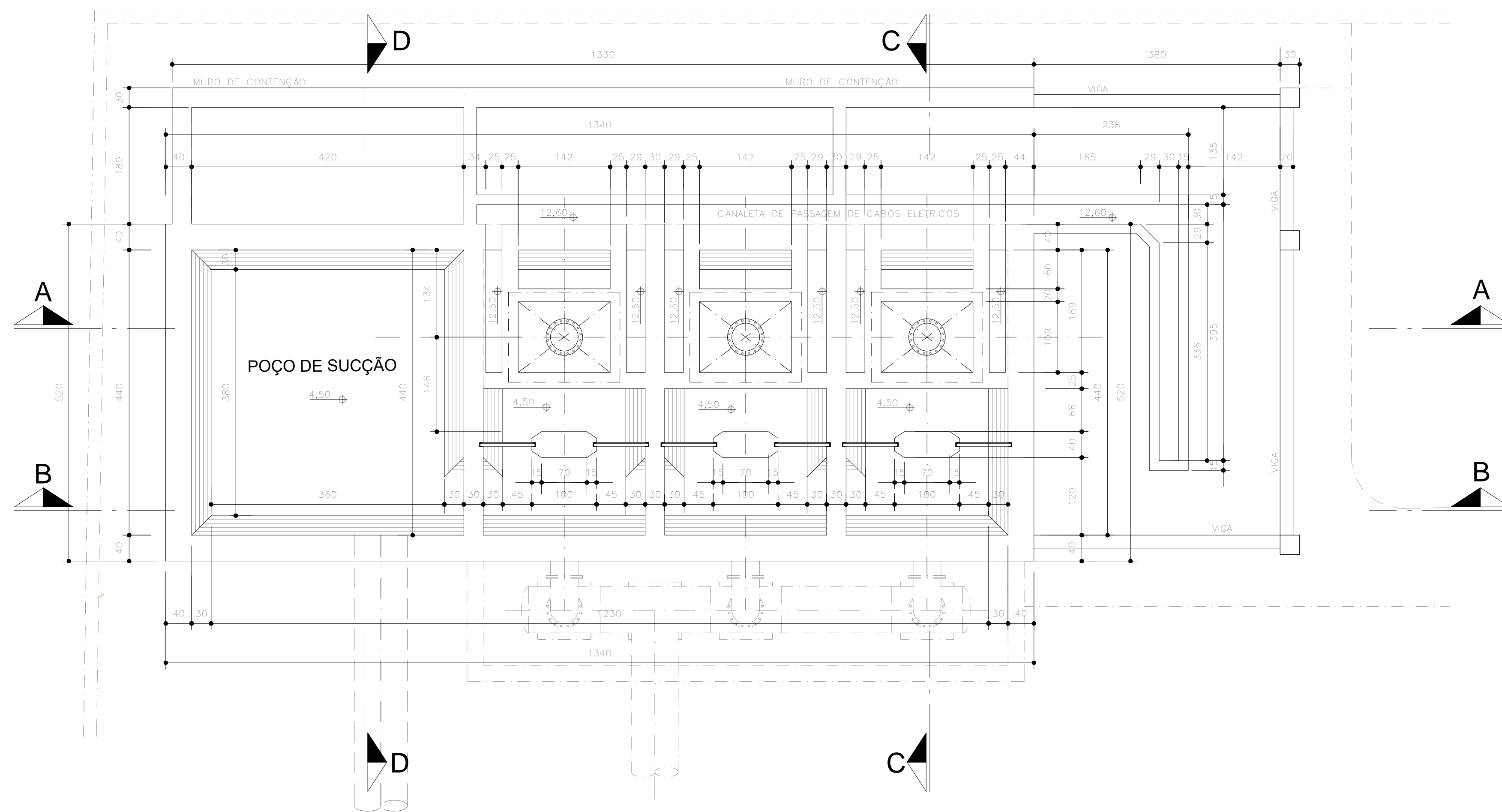
PLANTA BAIXA NO NÍVEL 12,60 ESCALA: 1/50
