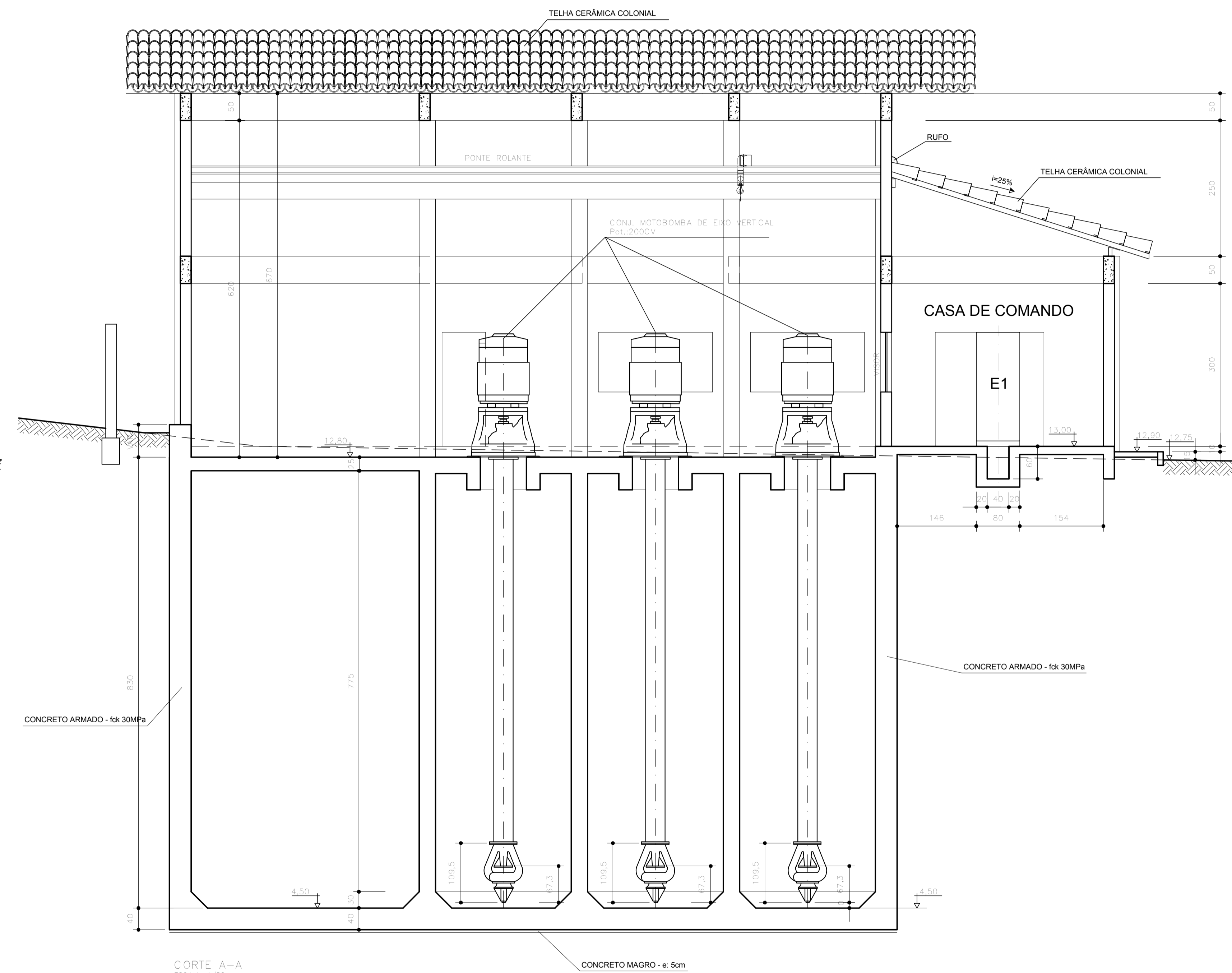
CORTE A-A ESCALA: 1/50
