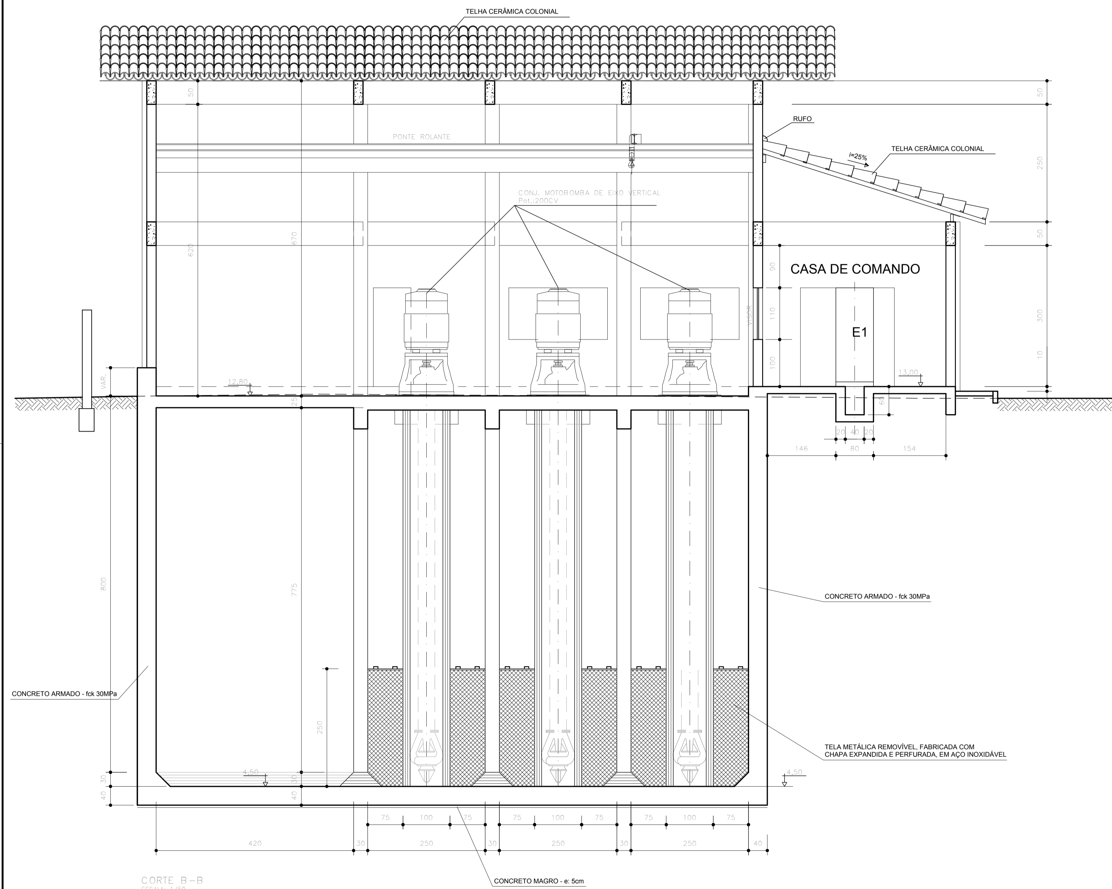
CORTE B-B ESCALA: 1/50
