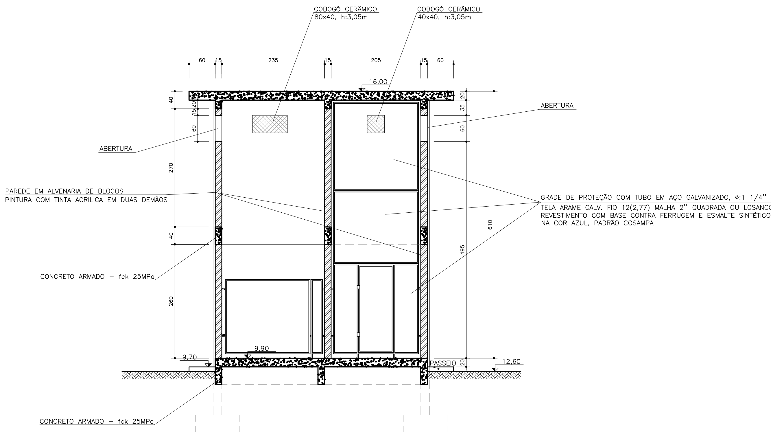
CORTE-A-A ESCALA 1/50
