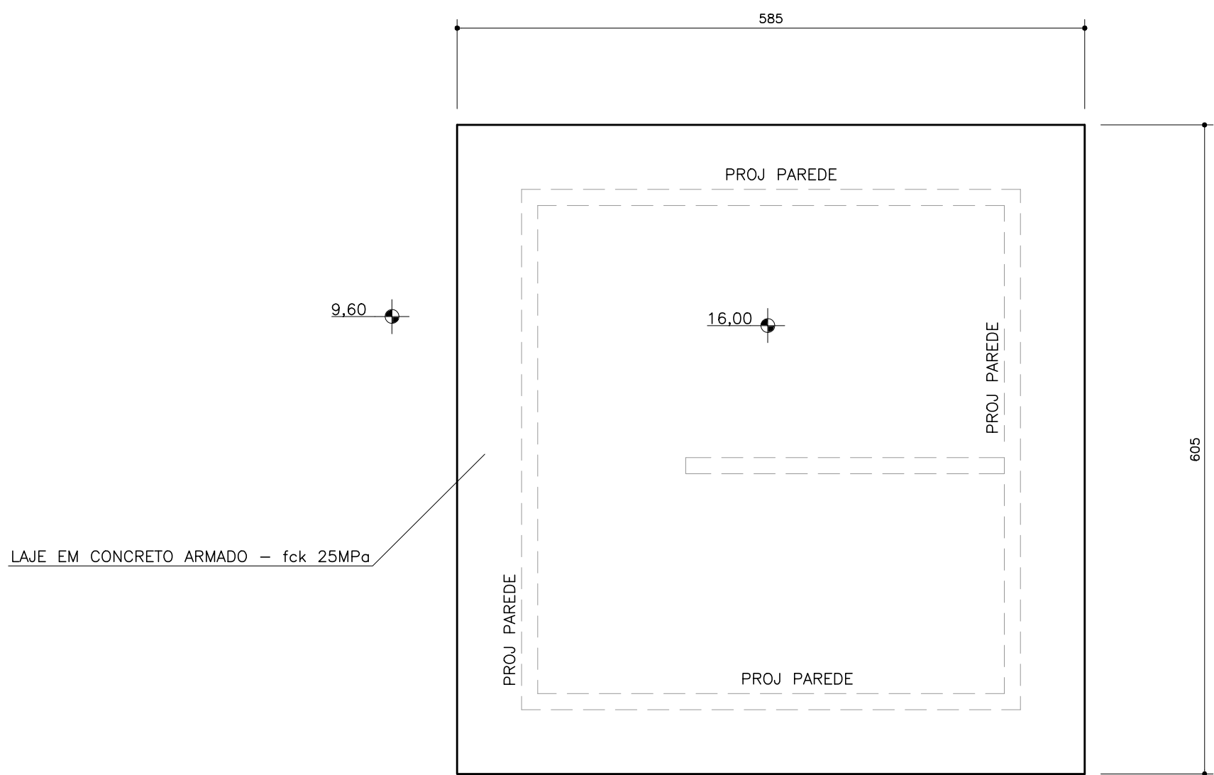
PLANTA DE COBERTURA ESCALA 1/50
