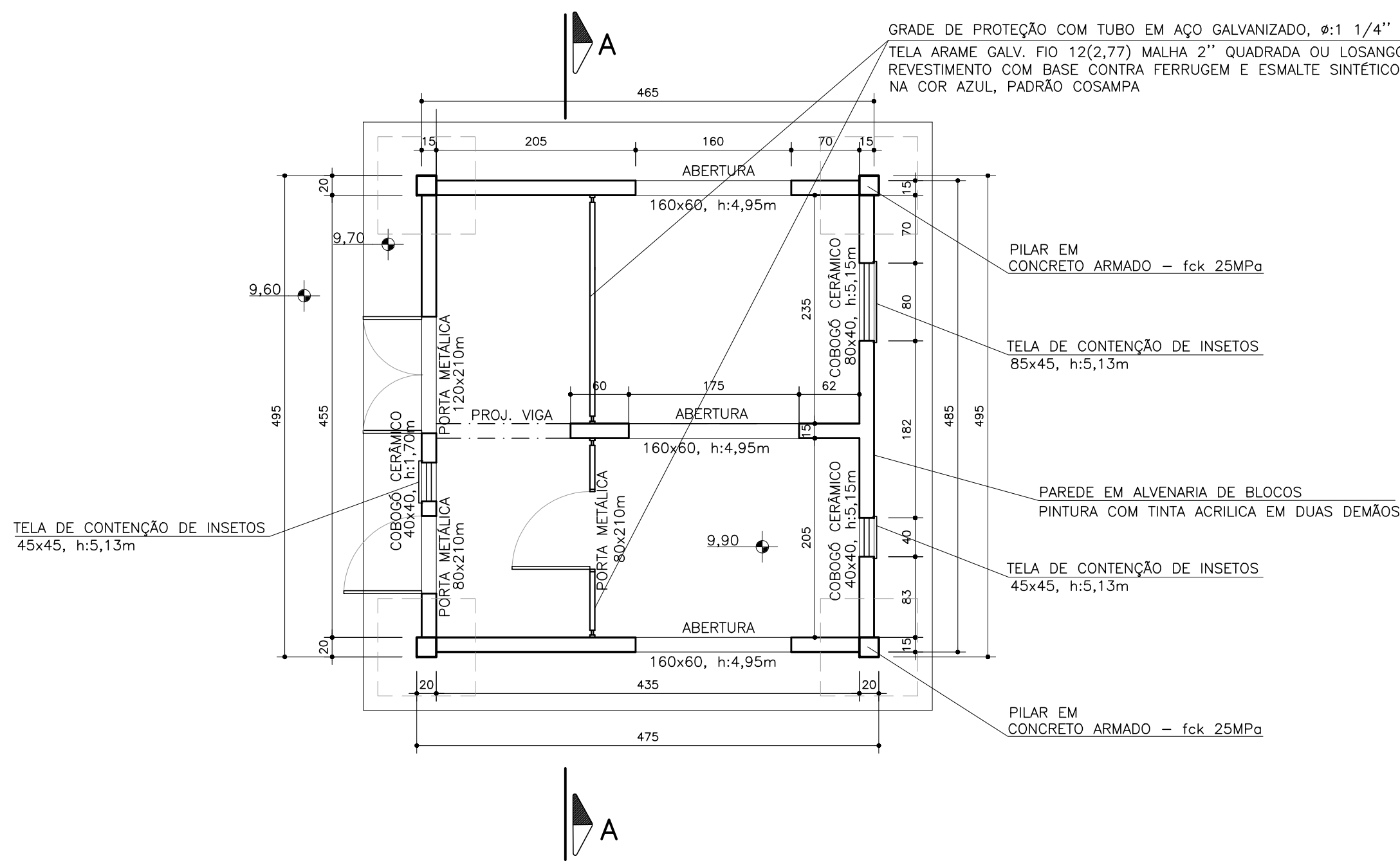
PLANTA BAIXA ESCALA 1/50
