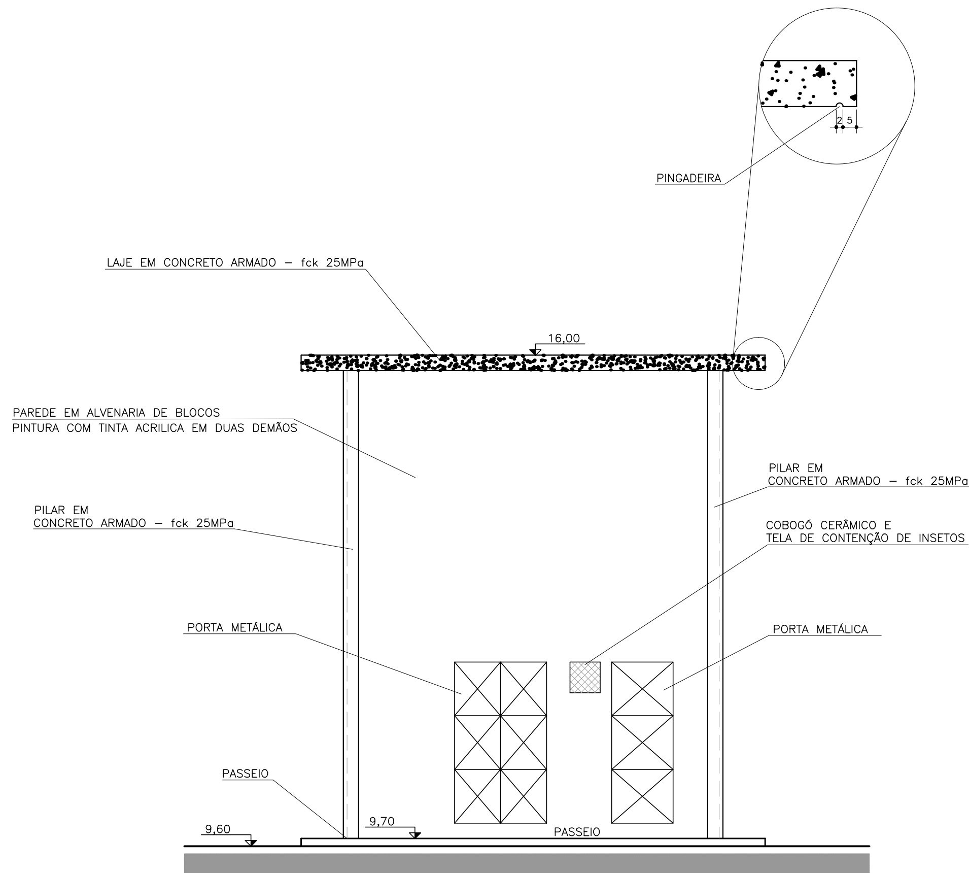
FACHADA ESCALA 1/50
