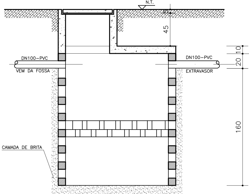
CORTE D-D
