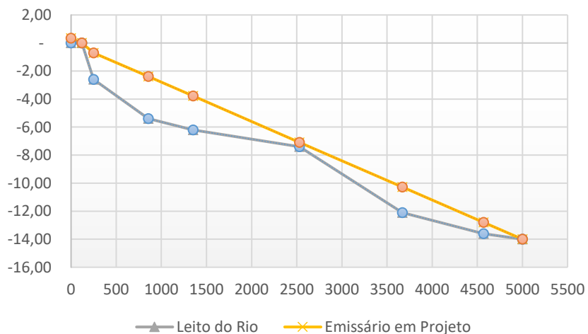
POSICIONAMENTO - Leito do Rio x Emissário em Projeto - Corte e Aterro
